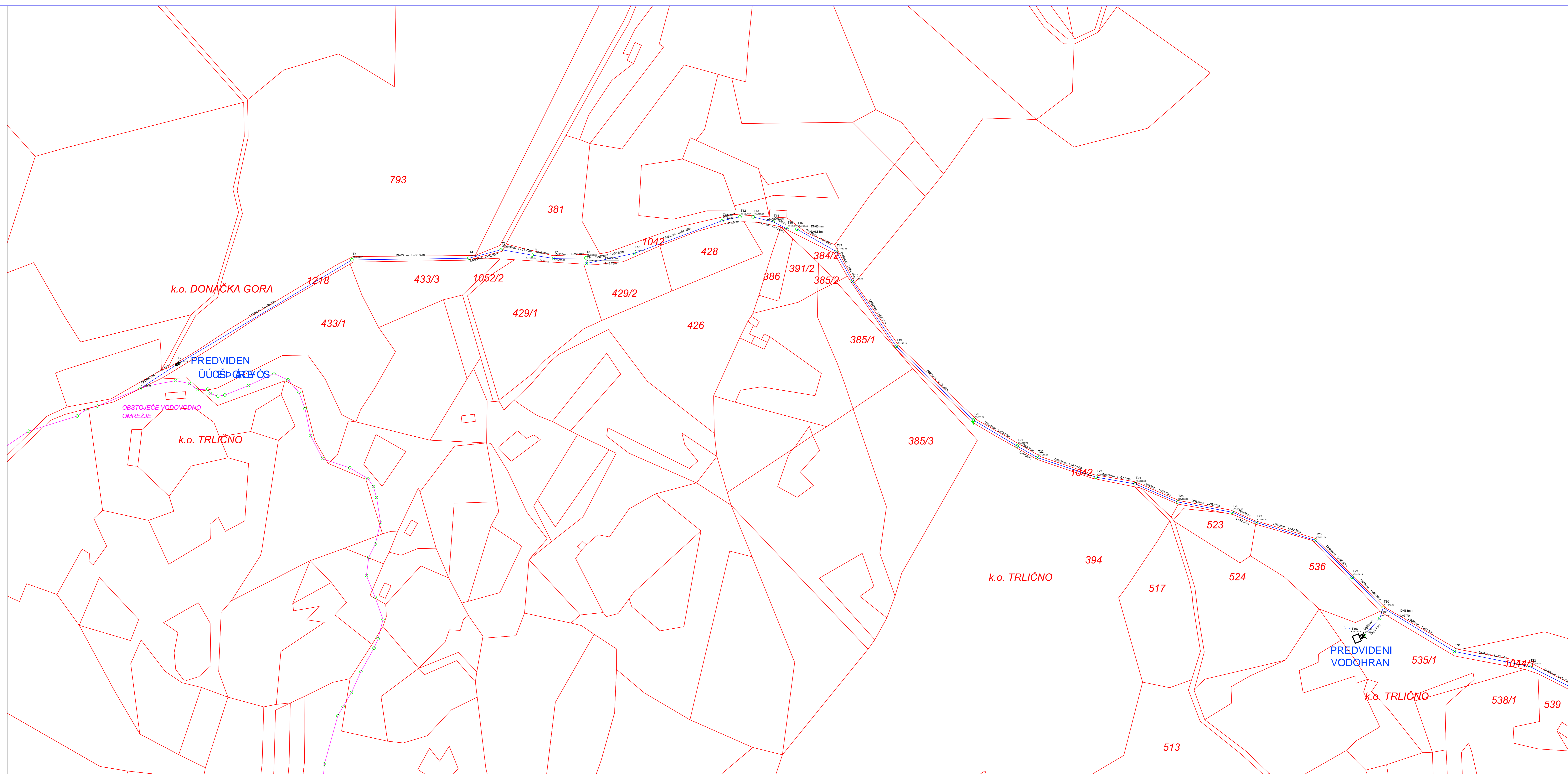
Situacija cevododa od T1 - T32 M 1:1000
